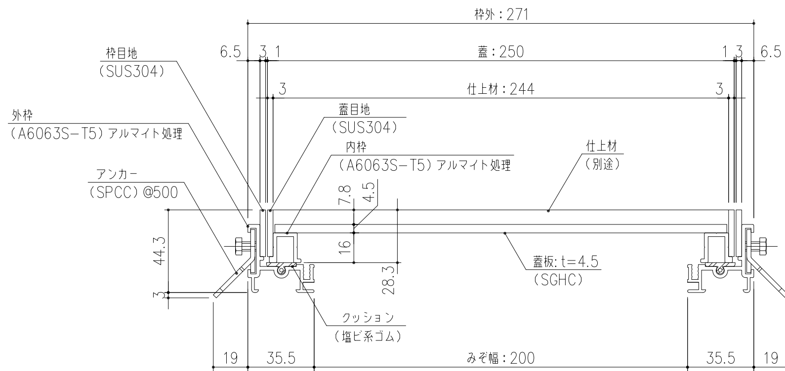
SP7-T4-25 断面詳細図 S=1/2 貼物用配線ピット蓋 ※荷重条件: 歩行用 (3.5KN/m 2 )
