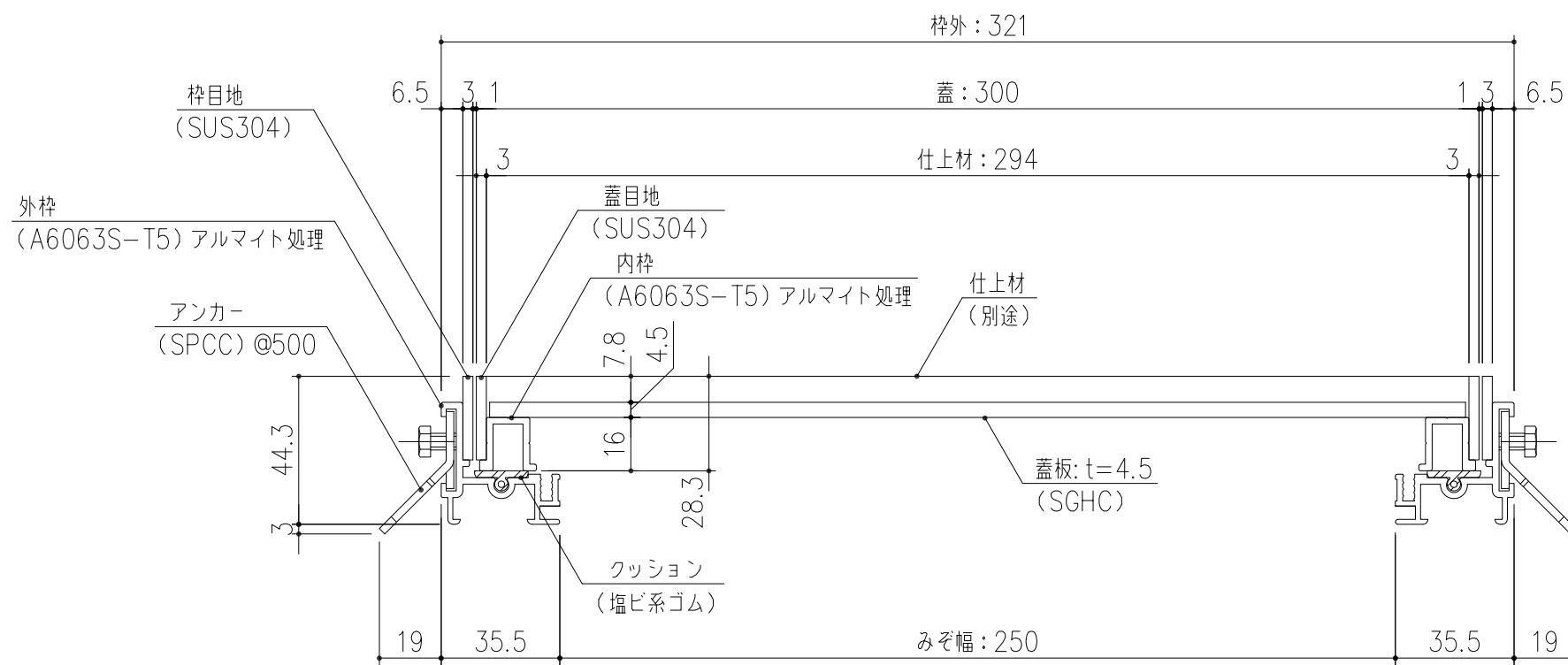
SP7-T4-30 断面詳細図 S=1/2 貼物用配線ピット蓋 ※荷重条件：歩行用 (3.5KN/m 2 )
