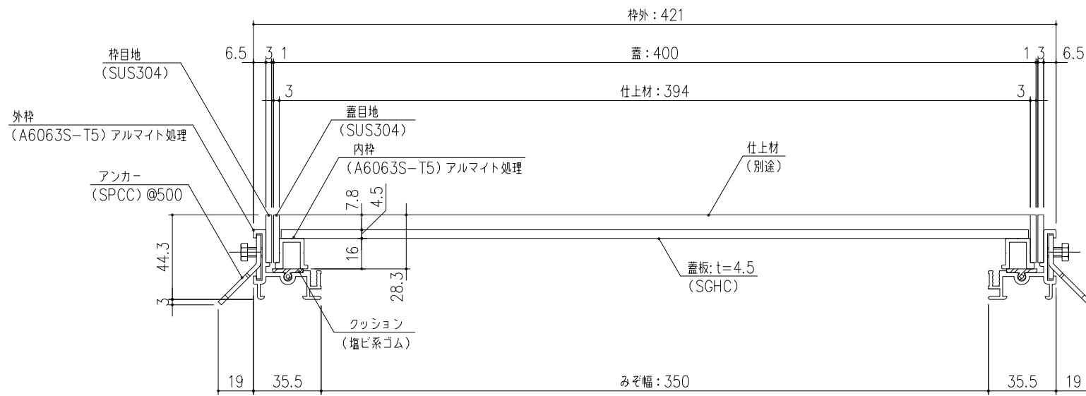
SP7-T4-40 断面詳細図 S=1/2 貼物用配線ピット蓋 ※荷重条件：歩行用 (3.5KN/m 2 )
