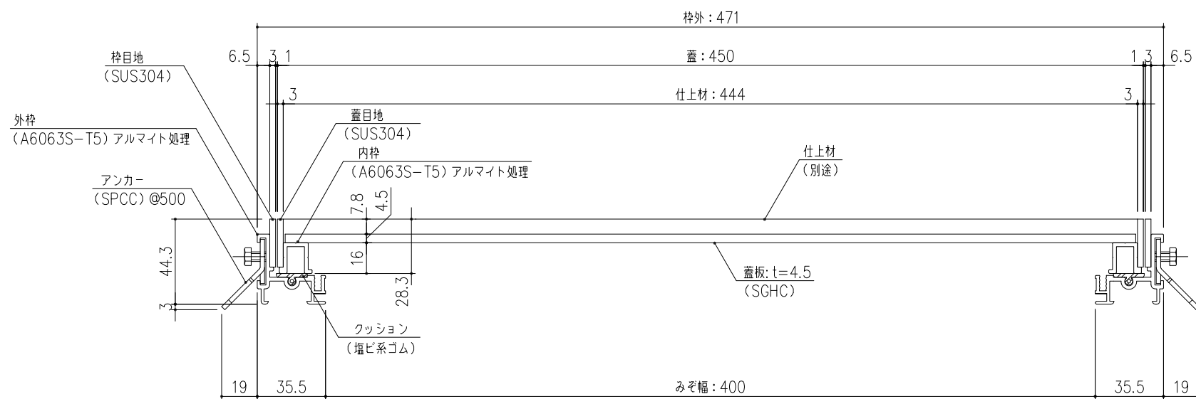
SP7-T4-45 断面詳細図 S=1/2 貼物用配線ピット蓋 ※荷重条件：歩行用 (3.5KN/m 2 )
