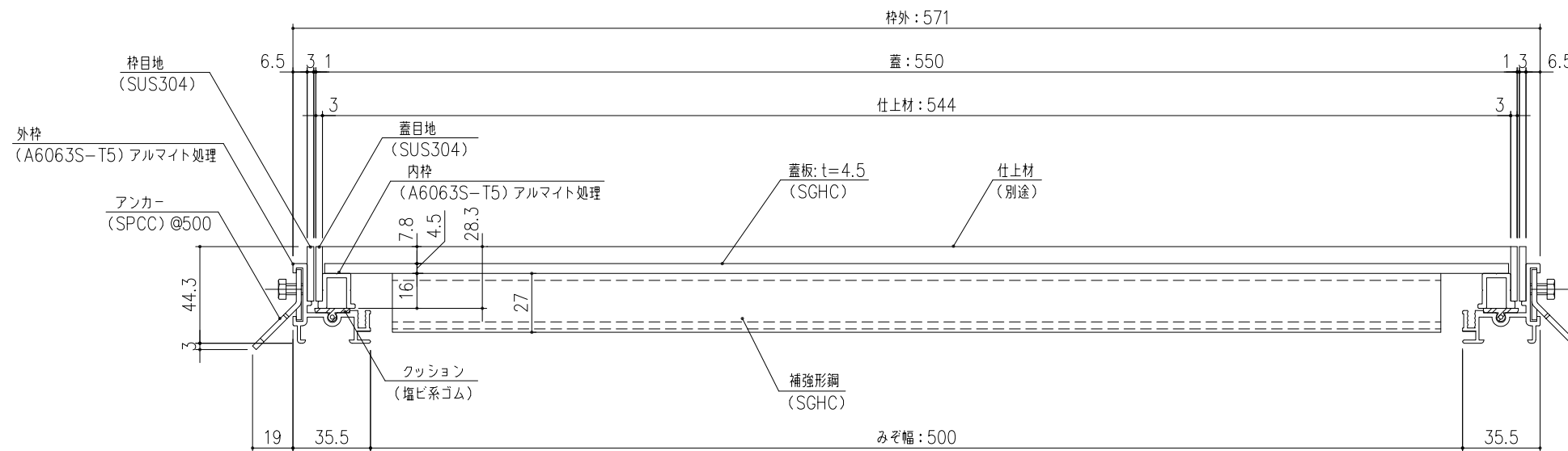
SP7-T4-55 断面詳細図 S=1/2 貼物用配線ピット蓋 ※荷重条件: 歩行用 (3.5KN/m 2 )
