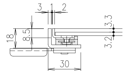
床仕上材の厚さ3.0mm用 SPE3-T3
