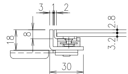
床仕上材の厚さ2.5mm用 SPE2.5-T3
