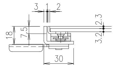
床仕上材の厚さ2.0mm用 SPE2-T3
