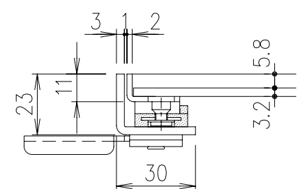
床仕上材の厚さ5.0mm用 SPE5-T3
