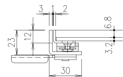
床仕上材の厚さ7.0mm用 SPE7-T3
