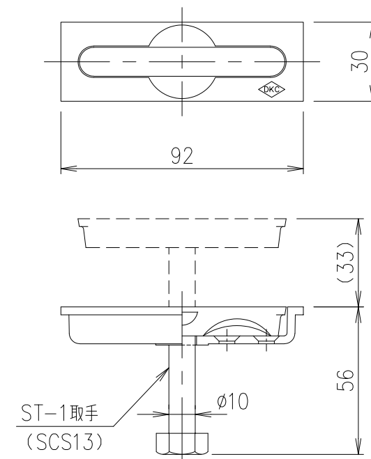
取手 (ST-1) 詳細図 S=1/2
