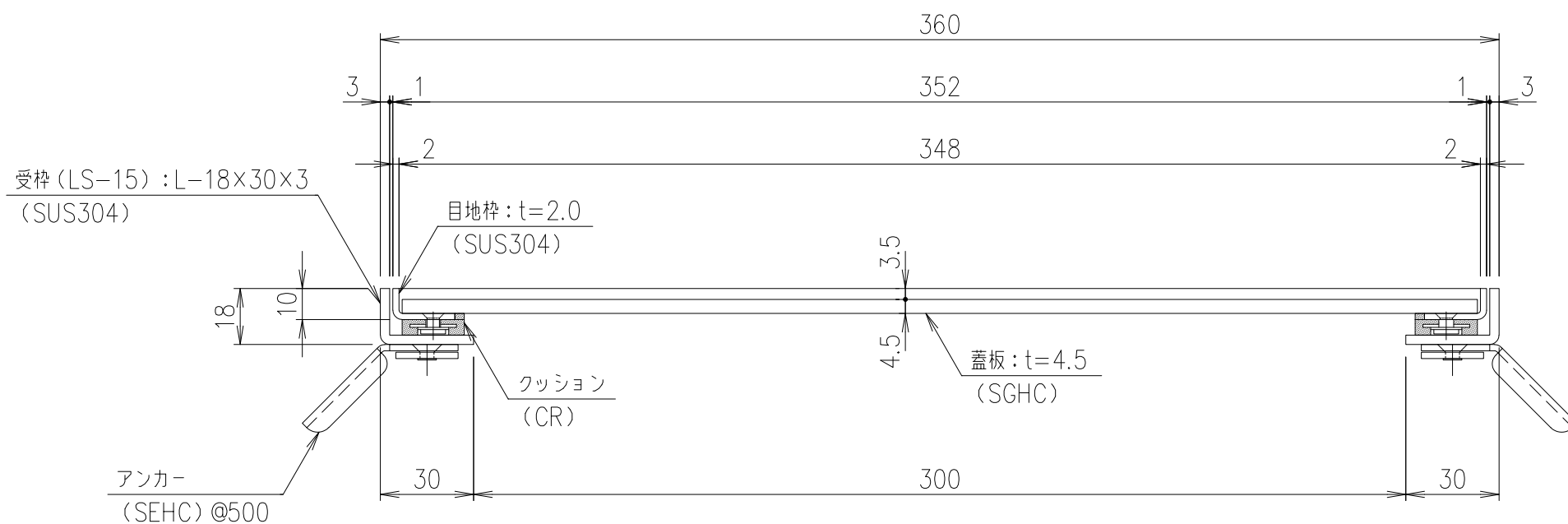
SPE3-T4-35 断面詳細図 S=1/2
