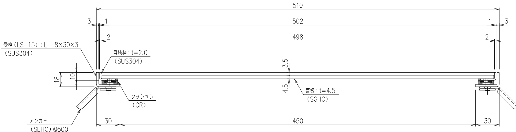
SPE3-T4-50 断面詳細図 S=1/2
