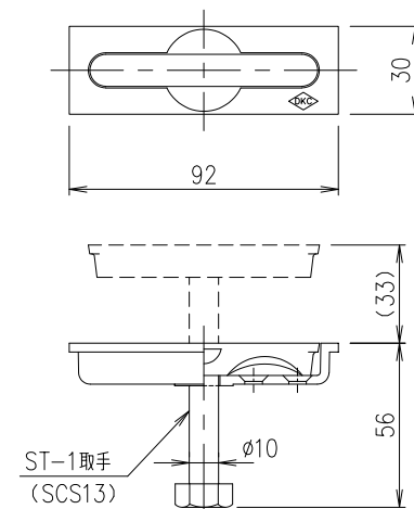
取手 (ST-1) 詳細図 S=1/2
