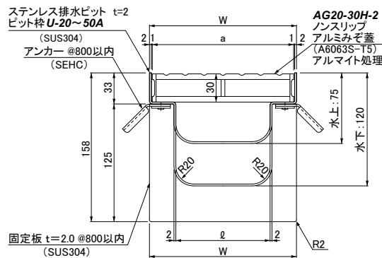
● U-A 断面詳細図
