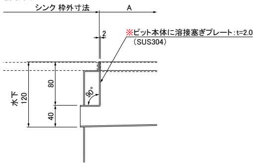
● U-A 断面詳細図
