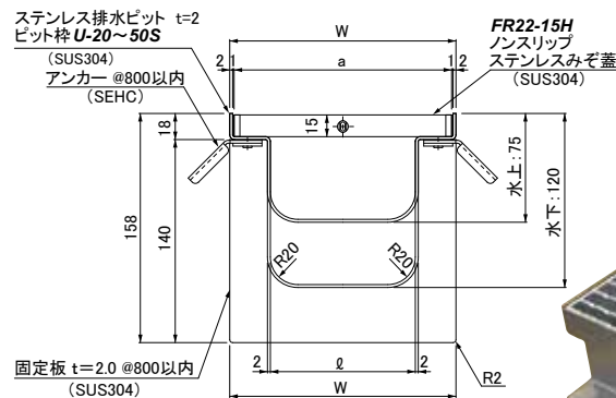
● U-S 断面詳細図
