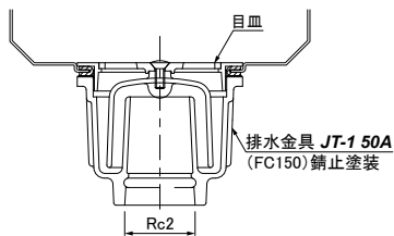
碗トラップ ソケットストレートタイプ 封水仕様(碗型トラップ式)
