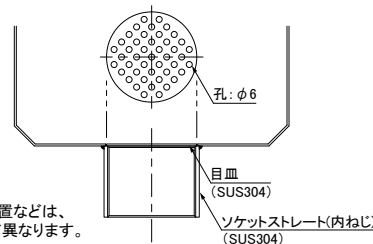
完全排水トラップ フランジタイプ 封水仕様(碗型トラップ脱着式) 【漏水による封水機能が損なわれないようにハンドルをきつく締めてください】
