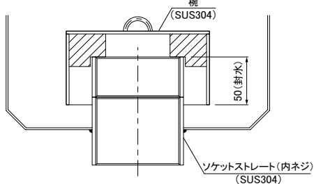
完全排水トラップ ソケットタイプ 封水仕様(碗型トラップ脱着式) 【漏水による封水機能が損なわれないようにハンドルをきつく締めてください】
