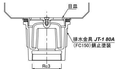
排水金具 JT-1 80A 封水仕様(碗型トラップ式) 【JT-1 80A は JT-1 50A の排水ネジ部のみを 80Aにした製品です】
