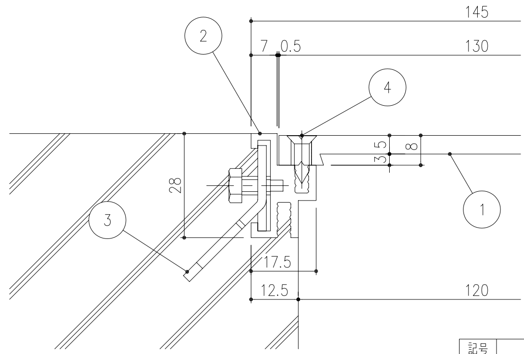
受枠部詳細 S=1/1
