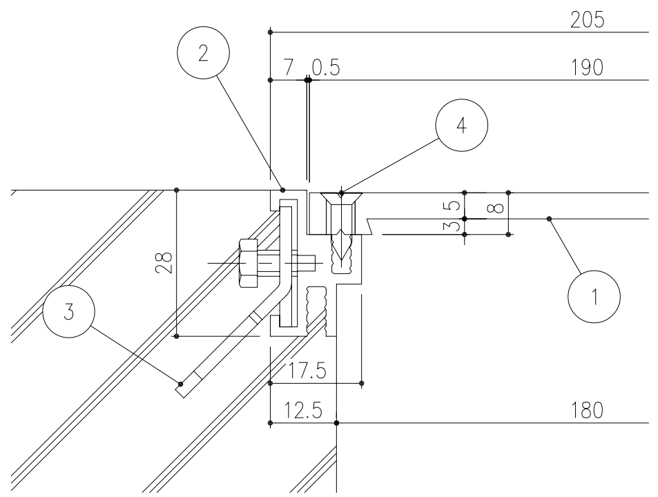
受枠部詳細 S=1/1
