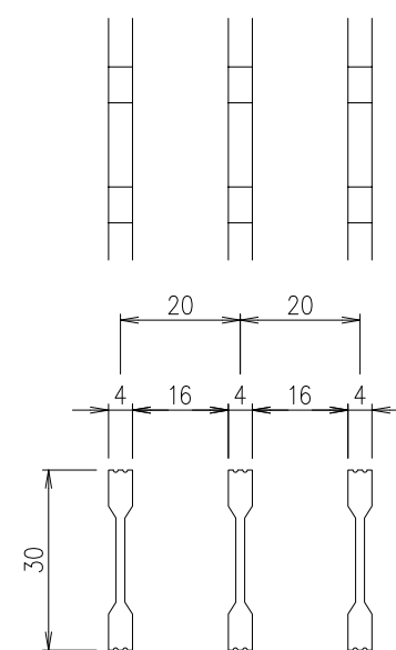
メインバーピッチ 詳細図 S=1/1 AGS20-3033-2
