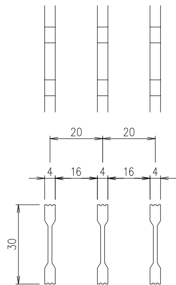
メインバーピッチ 詳細図 S=1/1 AGS20-3033-2
