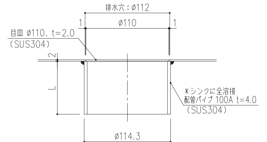
排水部 詳細図 S=1/3 ※L寸法を御指示下さい。
