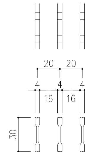
メインバー詳細図 S=1/2
