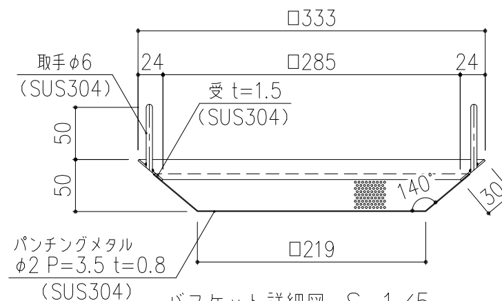
バスケット詳細図 S=1/5
