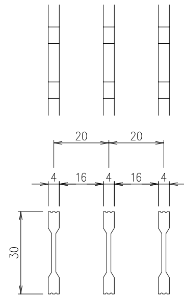
メインバーピッチ 詳細図 S=1/1 AGS20-3044-2
