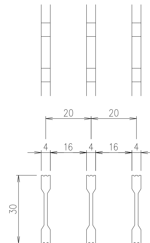
メインバーピッチ 詳細図 S=1/1 AGS20-3044-2
