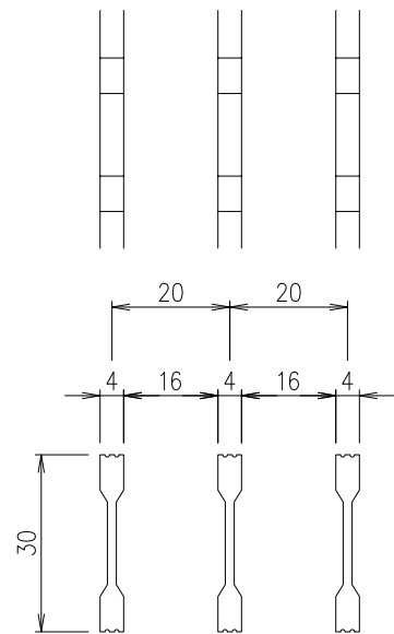
メインバーピッチ 詳細図 S=1/1 AGS20-3055-2
