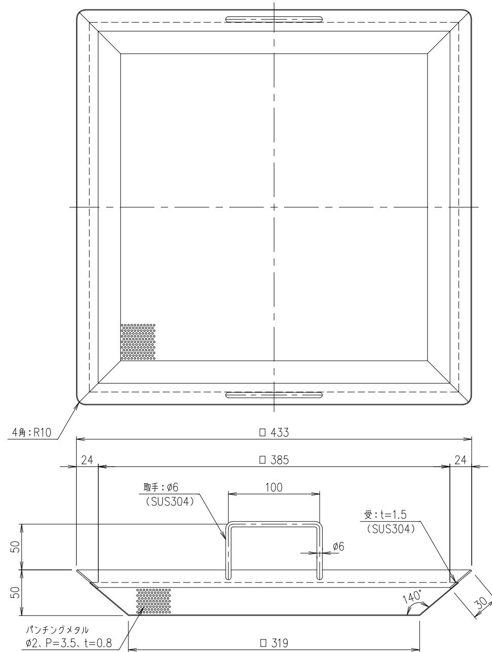
テーパバケット 詳細図 S=1/3
