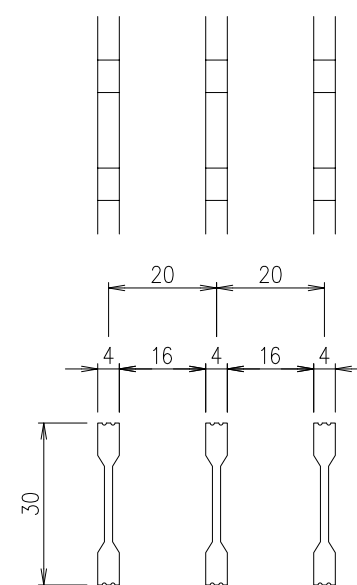
メインバーピッチ 詳細図 S=1/1 AGS20-3055-2
