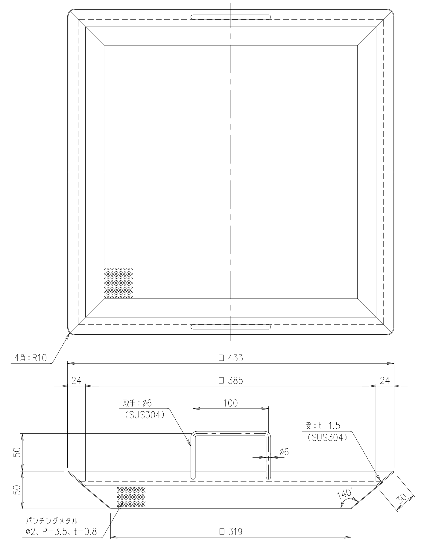
テーパーバスケット 詳細図 S=1/3
