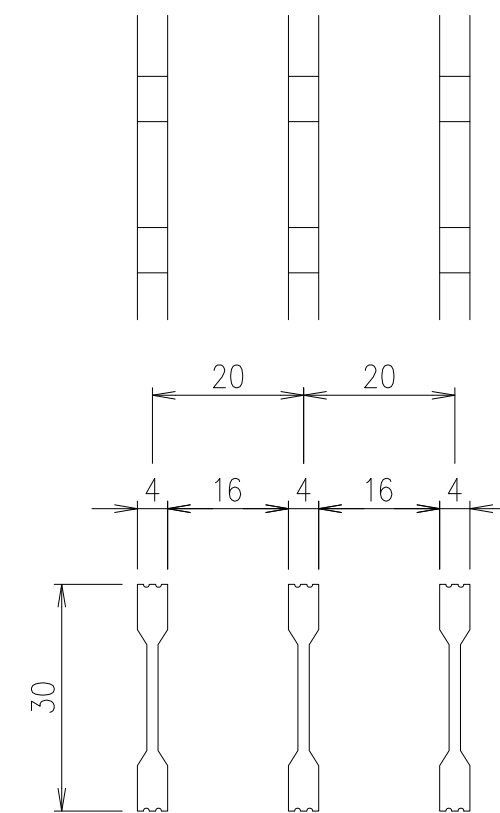
メインバーピッチ 詳細図 S=1/1 AGS20-3055-2
