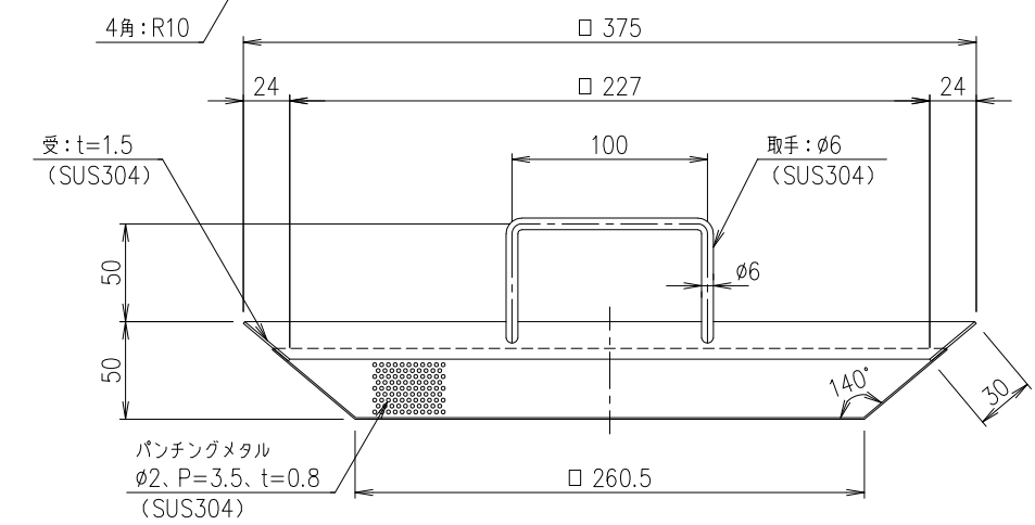
テーパースタック 詳細図 S=1/3
