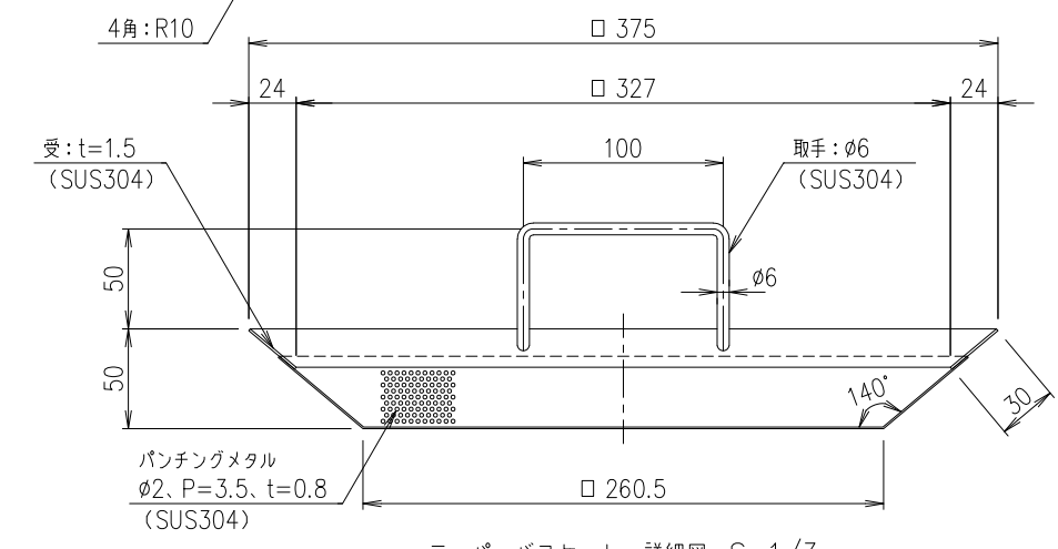
テーパースタケット 詳細図 S=1/3
