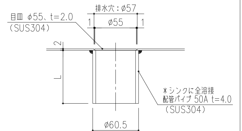
排水部 詳細図 S=1/3 ※寸法を御指示下さい。
