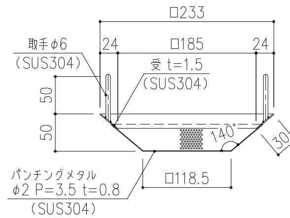
バスケット詳細図 S=1/5
