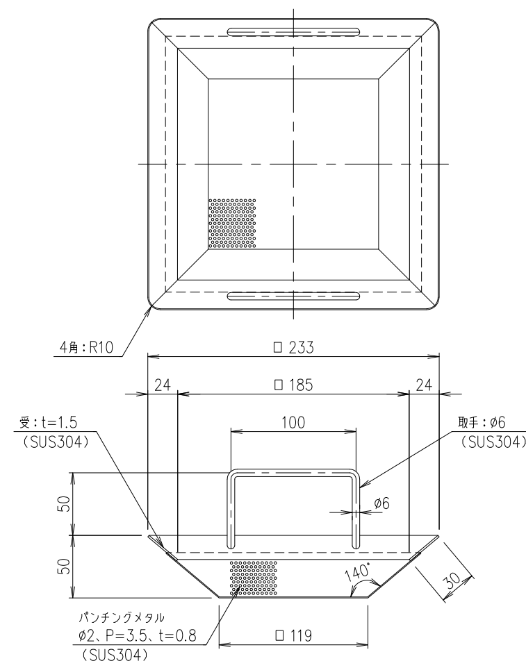
テーパーバスケット 詳細図 S=1/3
