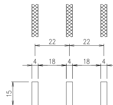
メインバーピッチ詳細図 S=1/1 FRM22-1530
