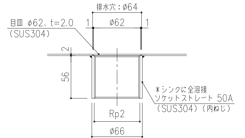
排水部 詳細図 S=1/3
