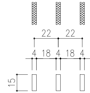
メンバー詳細図 S=1/2
