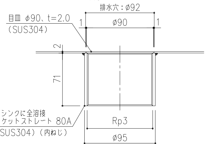
排水部 詳細図 S=1/3
