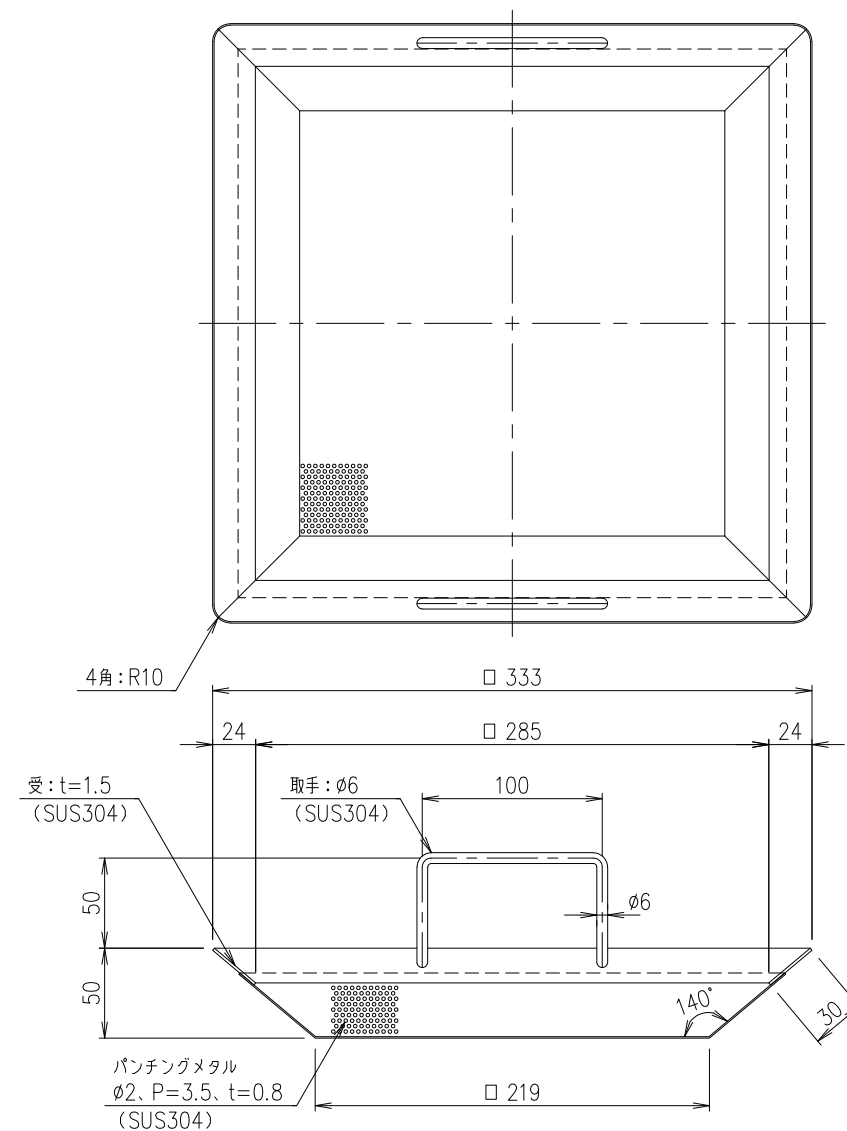
テーパーバスケット 詳細図 S=1/3
