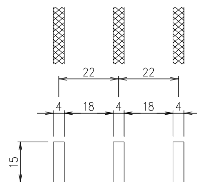
メインバーピッチ 詳細図 S=1/1 FRM22-1540
