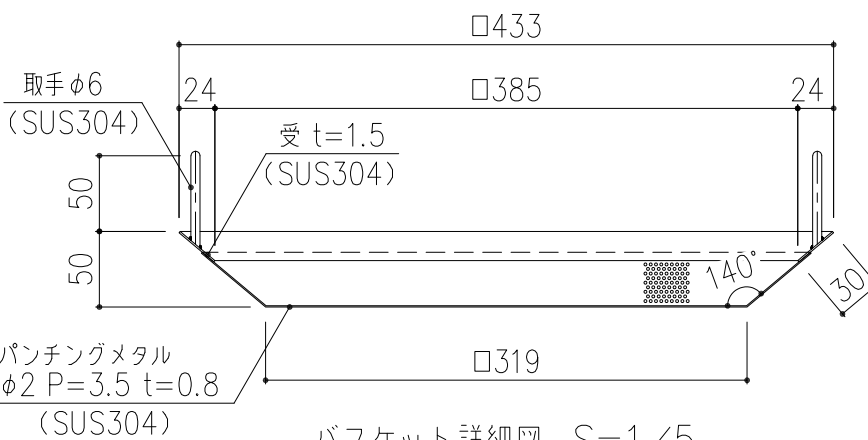
バスケット詳細図 S=1/5
