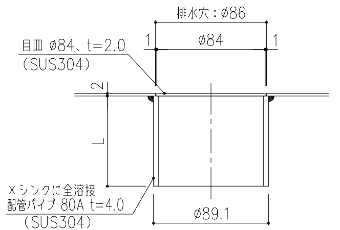
排水部 詳細図 S=1/3 ※L寸法を御指示下さい。
