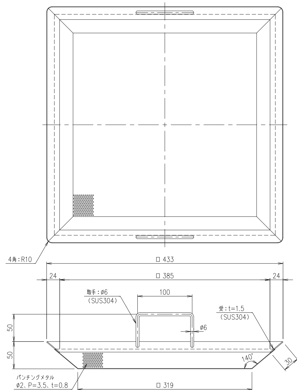
テーパーバスケット 詳細図 S=1/3
