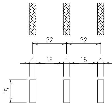
メインバーピッチ 詳細図 S=1/1 FRM22-1550
