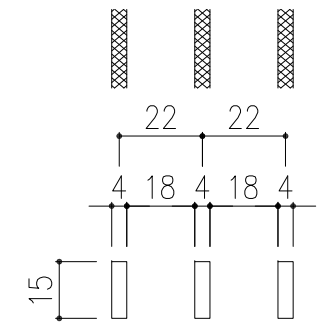
メインバー詳細図 S=1/2
