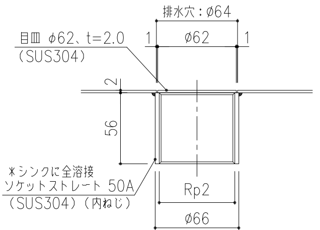
排水部 詳細図 S=1/3
