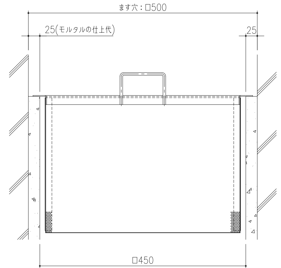
施工例
