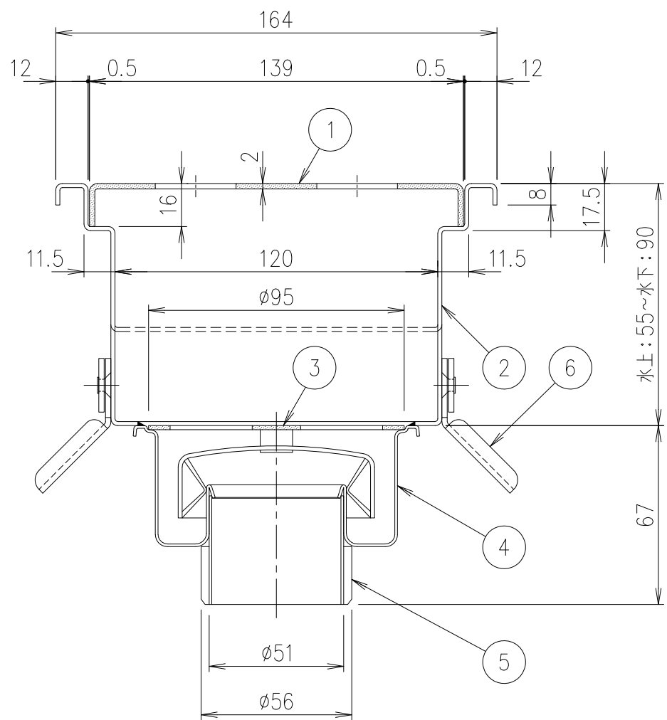
断面詳細図 S=1/2
