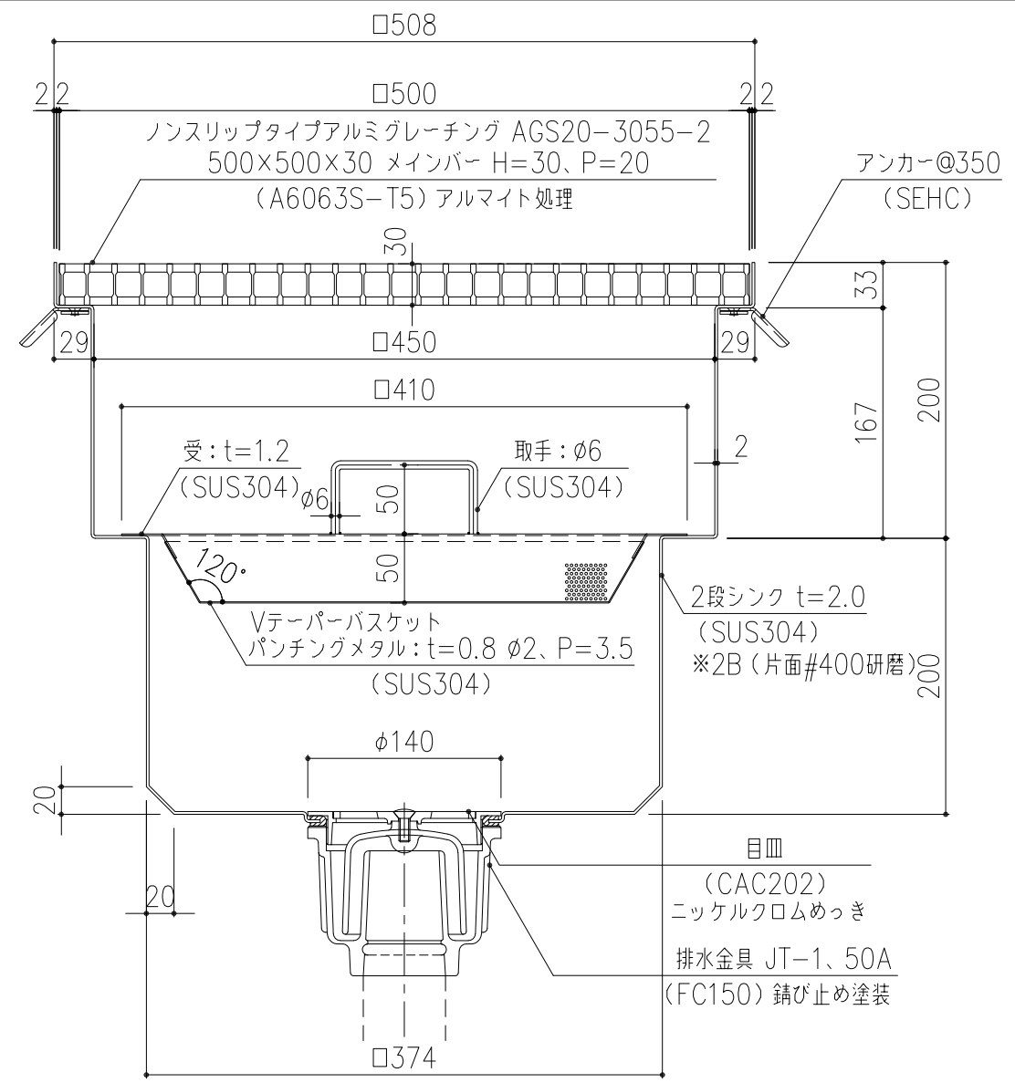
2段シンク 断面詳細図 S=1/5 蓋：AGS20-3055-2、排水金具JT-1、50A
