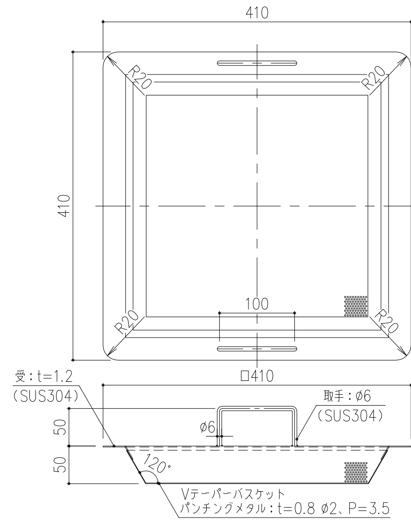
Vテーパーバスケット 断面詳細図 S=1/5
