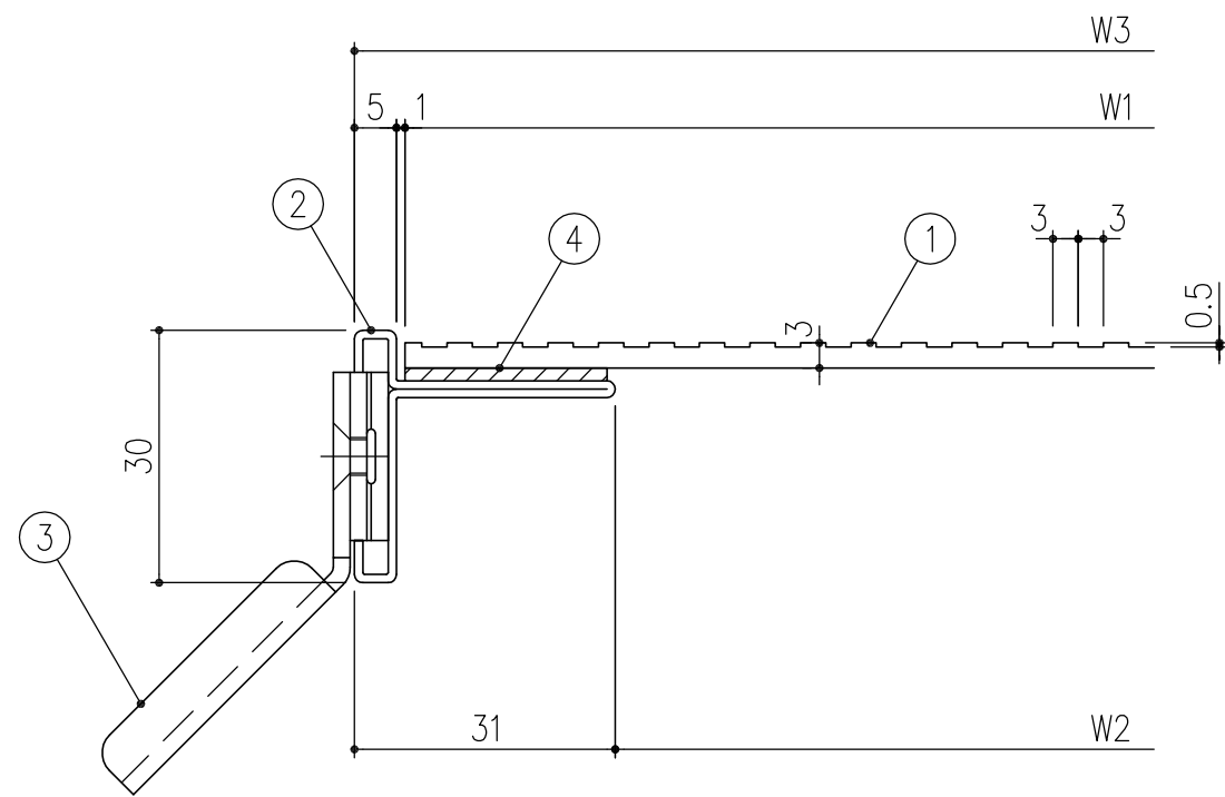
SP-2N (LP-4枠) 断面詳細図 S=1/1
