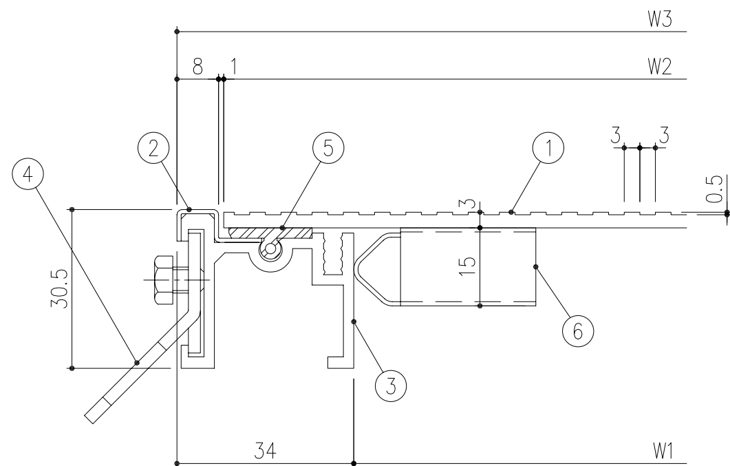
SP-2N (SFK-2枠) 断面詳細図 S=1/1
