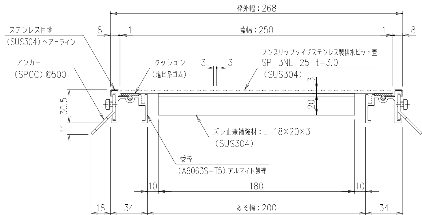
SP-3NL-25 断面詳細図 S=1/2
