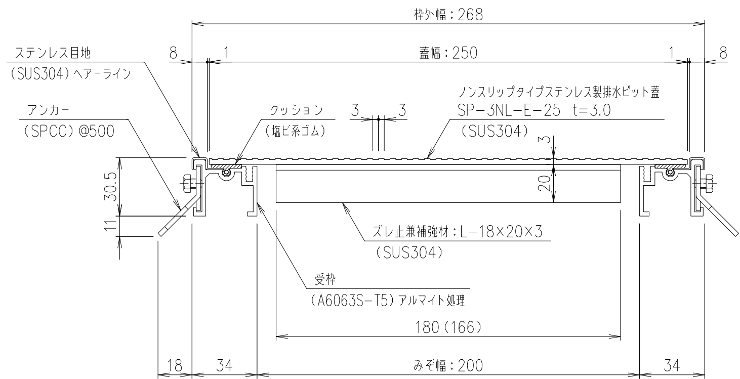
SP-3NL-E-25 断面詳細図 S=1/2 ノンスリップタイプステンレス製排水ピット蓋
