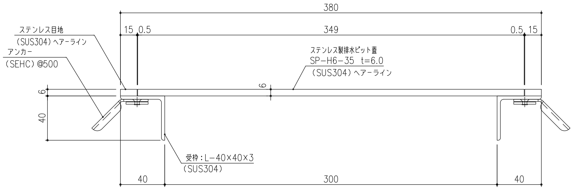
断面詳細図 S=1/2
