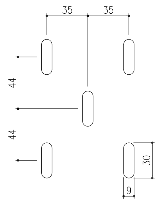
排水穴詳細図 S=1/2
