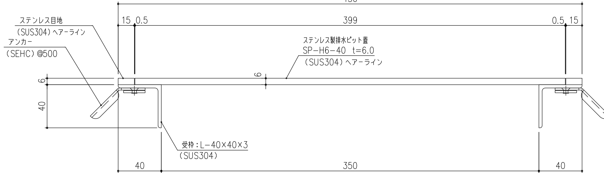
断面詳細図 S=1/2
