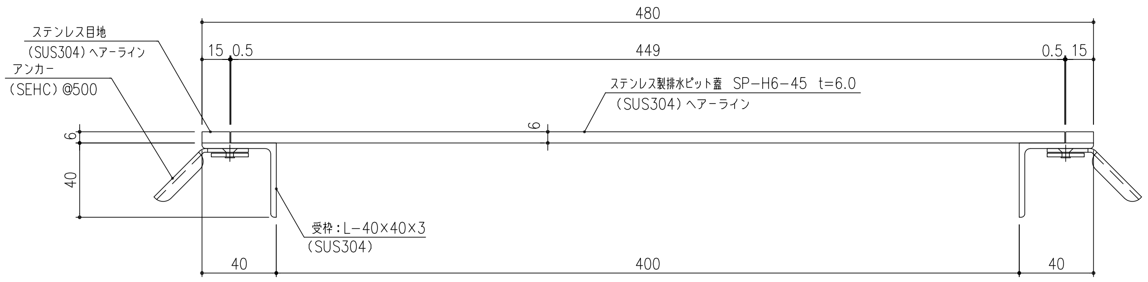
断面詳細図 S=1/2
