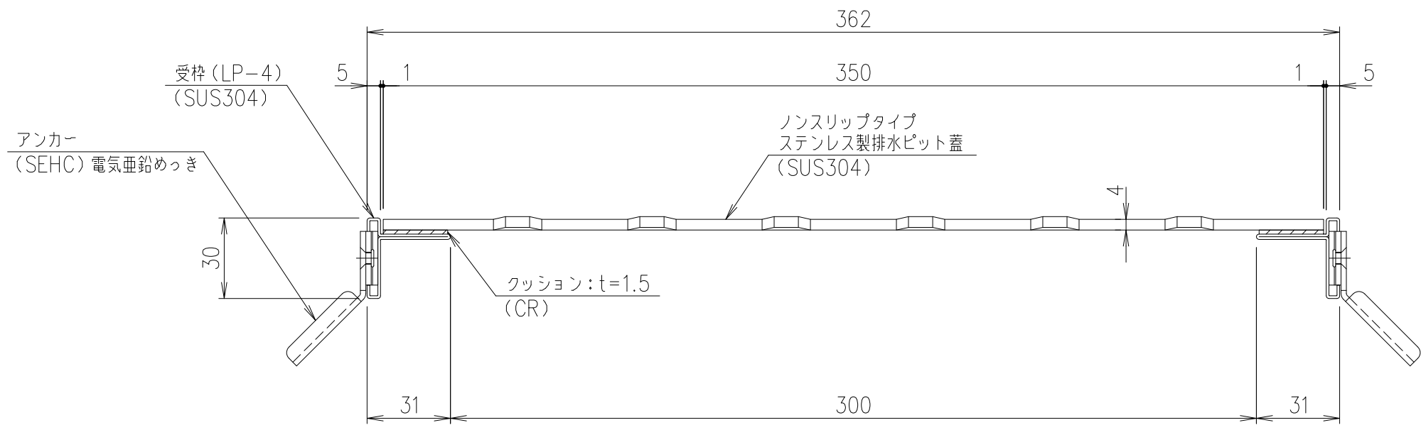
断面詳細図 S=1/2
