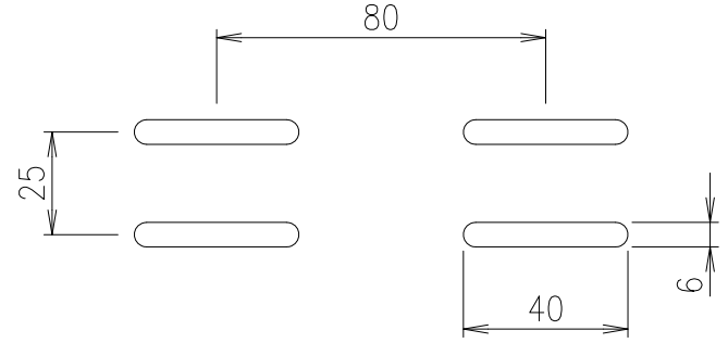
排水穴 詳細図 S=1/2
