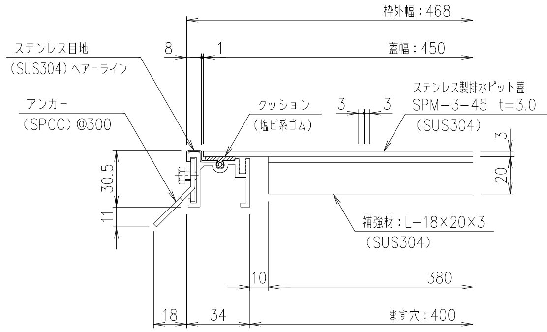
SPM-3-45 断面詳細図 S=1/2 ステンレス製排水ピット蓋
