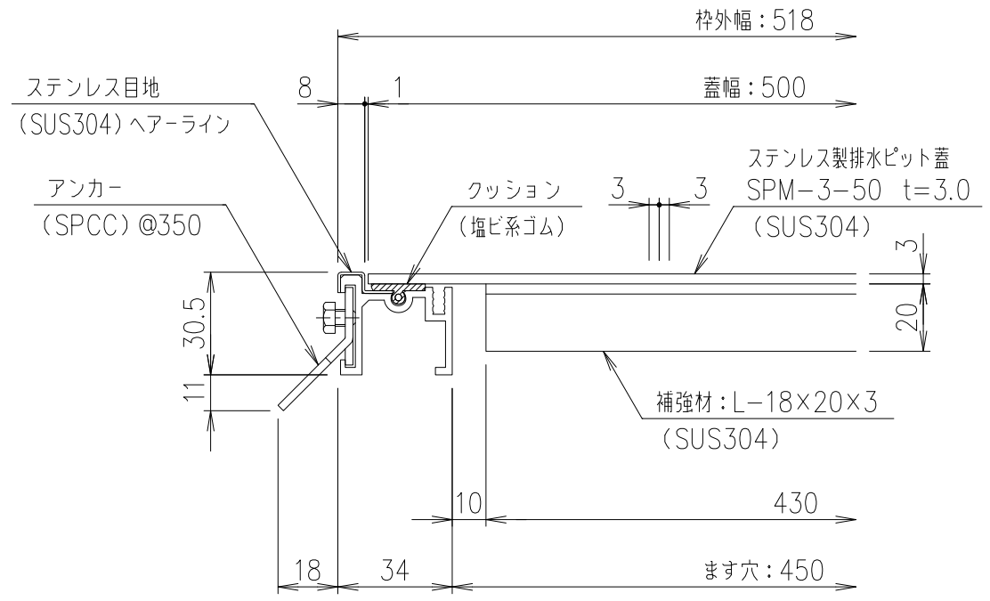
SPM-3-50 断面詳細図 S=1/2 ステンレス製排水ピット蓋
