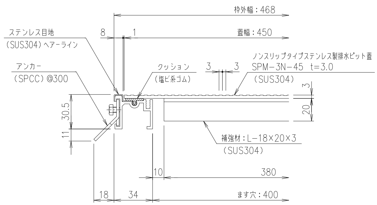
SPM-3N-45 断面詳細図 S=1/2 ノンスリップタイプステンレス製排水ピット蓋
