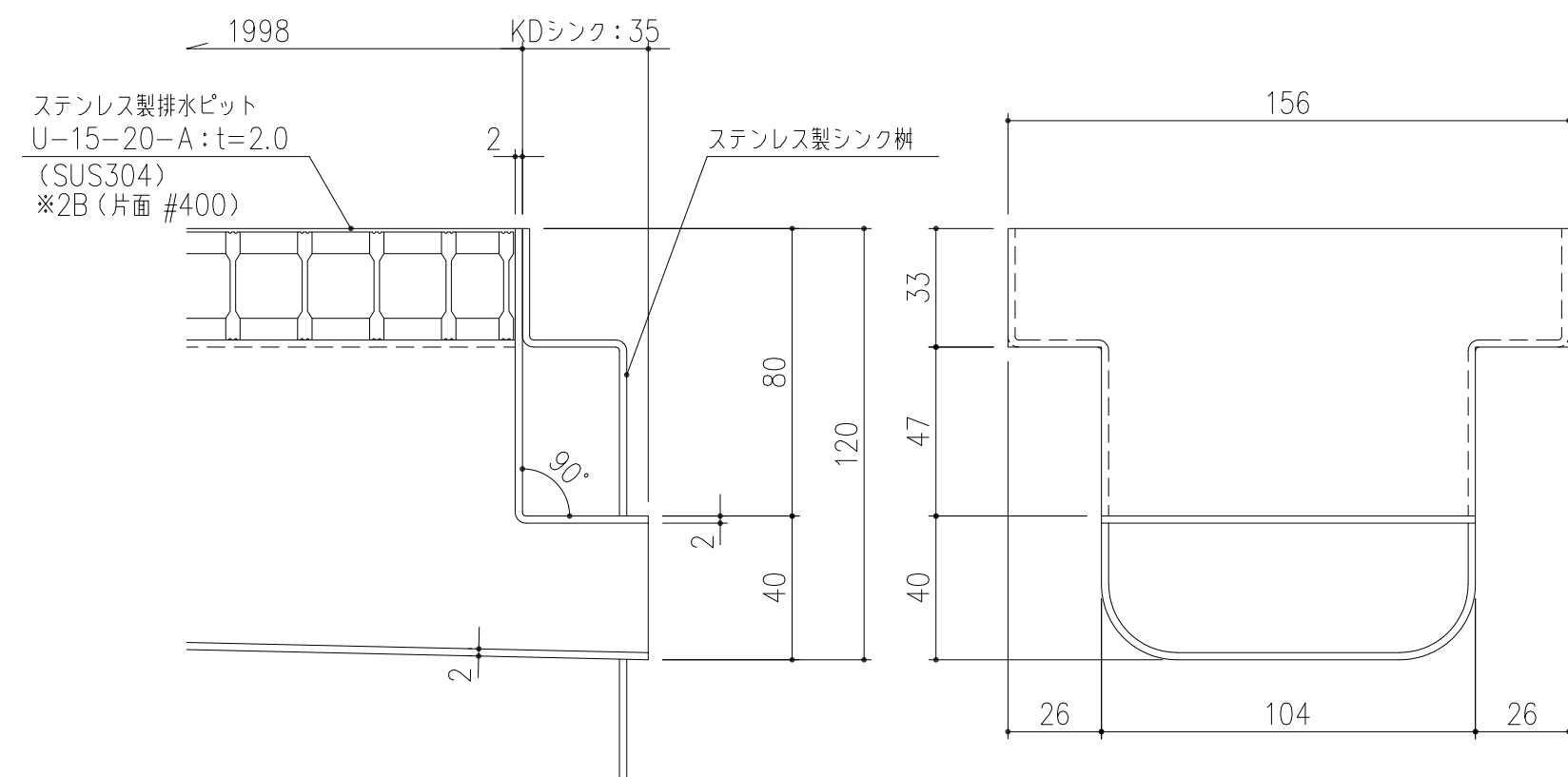
接続部詳細図 S=1/2
