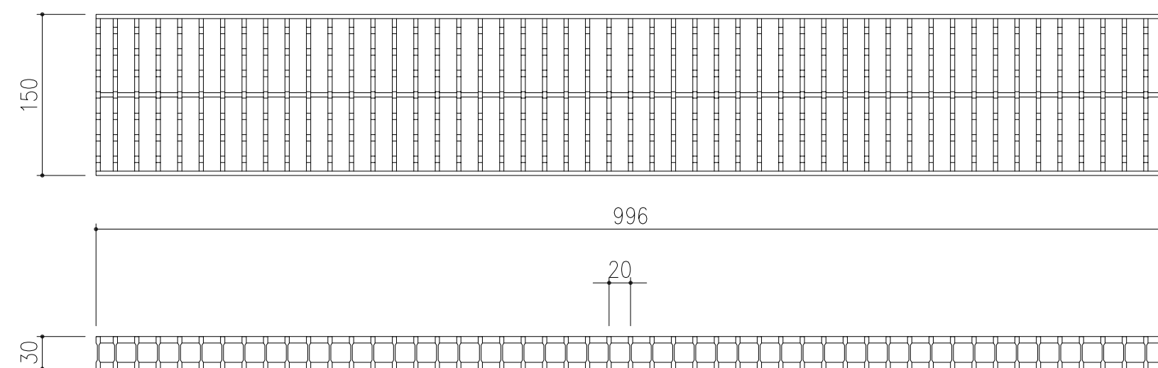
AG20-3015-2 詳細図 S= /5
