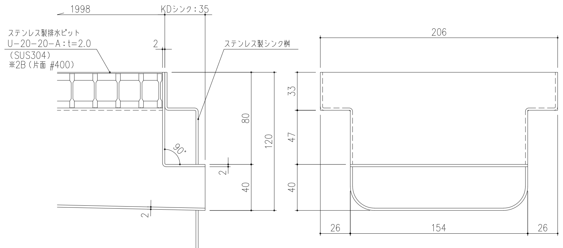
接続部詳細図 S=1/2
