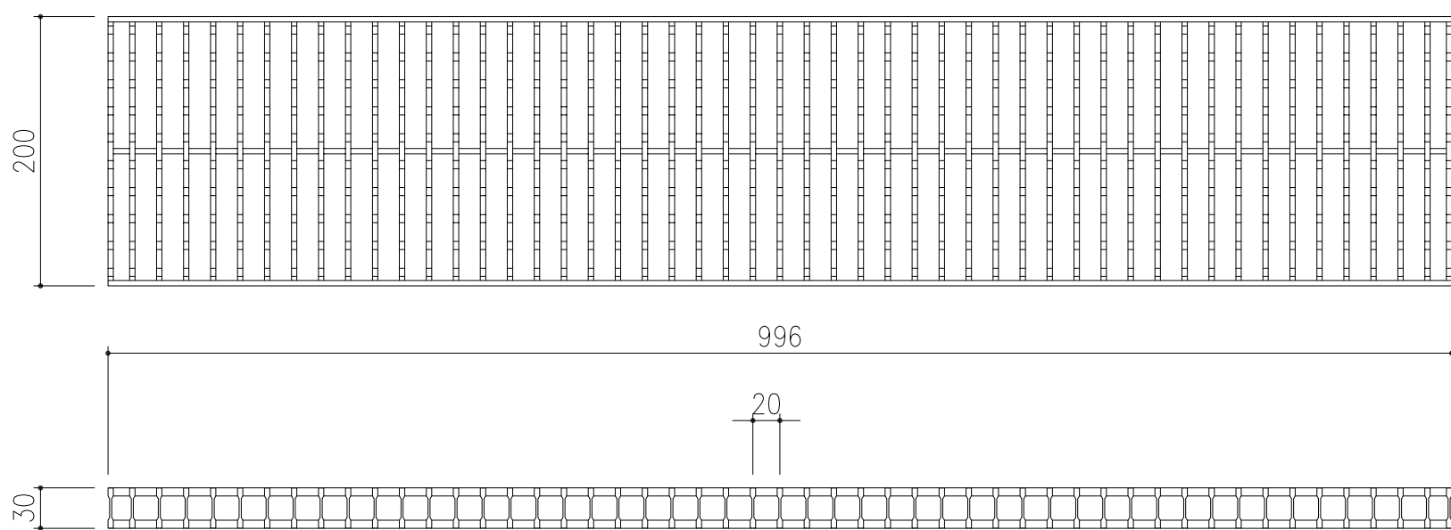
AG20-3020-2 詳細図 S= /5
