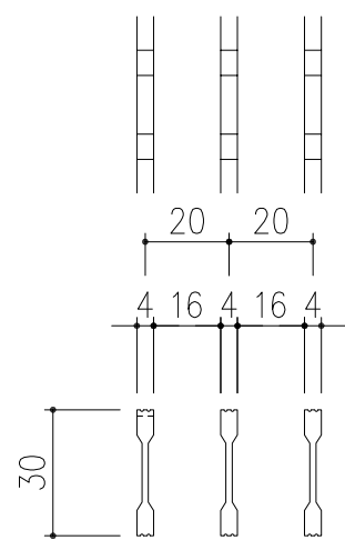
メンバーピッチ詳細図 S=1/2
